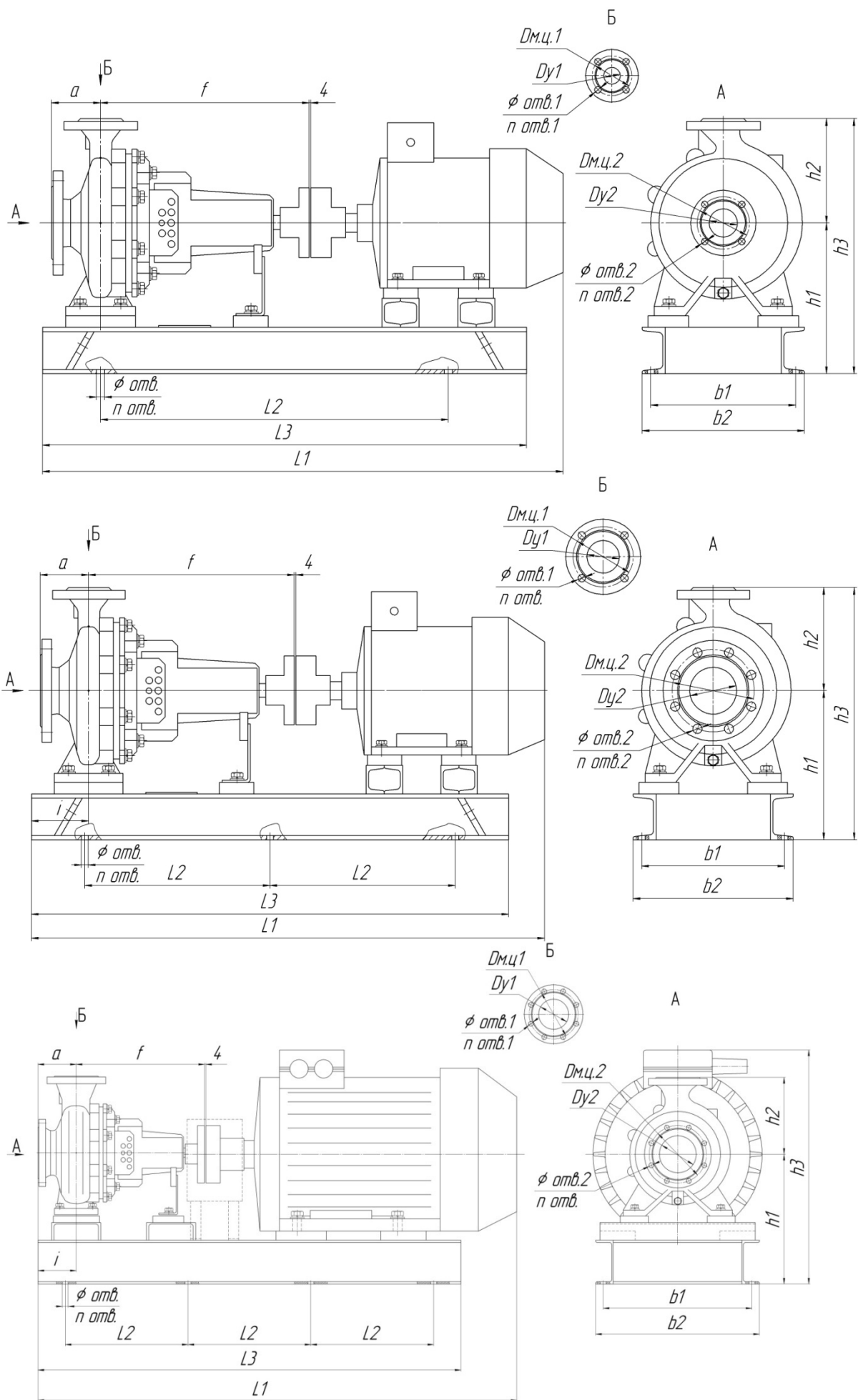
Рис 6. Габаритные и присоединительные размеры "Иртыш" – ЦНК.
